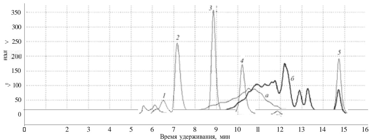
Рис. 3. Хроматограммы образцов ОА, УФ и стандартов реперных соединений (детектирование при 214 им). Обозначения: а — образец ОА; б — образец УФ; реперные соединения: 1 — димер БСА (130 кДа), 2 — БСА (65 кДа), 3 — лактальбумин (14 кДа), 4 — апротинин (6,5 кДа), 5 — триптофан (0,2 кДа).
