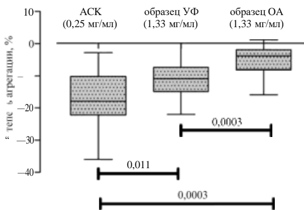
Рис. 4. Значимость различий (результаты одновыборочного теста Вилкоксона) между парами образцов для степени агрегации тромбоцитов.
